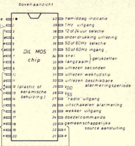
Fig. 6. Aansluitgegevens van het 40-pens klok IC.
